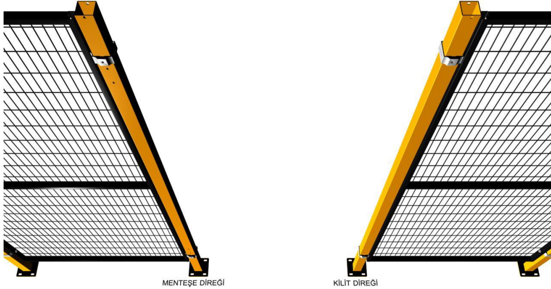
SOL AÇILIMLI KAPI İÇİN DİREK KONUMLANDIRILMASI
