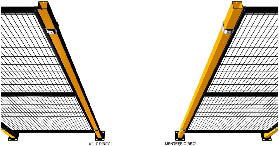
SAĞ AÇILIMLI KAPI İÇİN DİREK KONUMLANDIRILMASI
