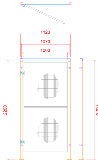
SİSTEM ÖLÇÜLERİ
